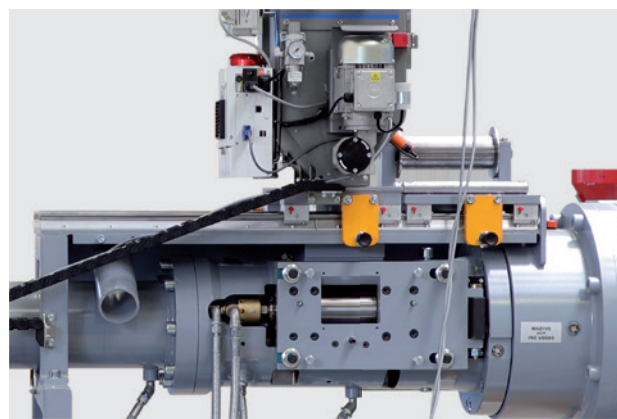
Detal systemu przesuwu leja i podajnika taśmowego
